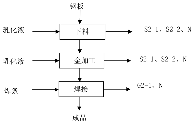
图 2-3-2 非标金属结构件工艺流程及产污环节示意图
