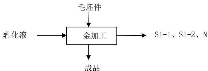
图 2-3-1 五金加工件生产工艺流程及产污环节示意图
